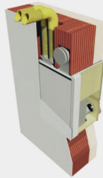
WANDINTEGRIERTER EINBAU U 2 MIT KANALANSCHLUSS
