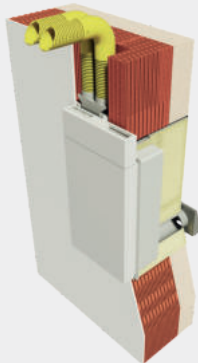
UNTERPUTZAUSFÜHRUNG MIT KANALANSCHLUSS
